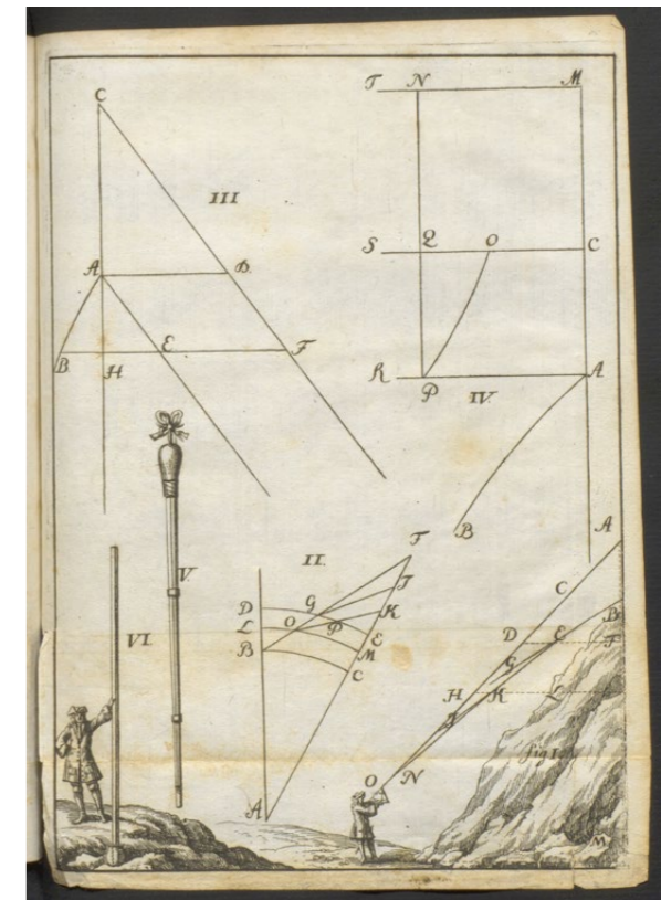
Abb. 2: Bild der Instrumente, die Scheuchzer während seiner Alpenreisen benutzte, wie zum Beispiel den Wanderstock mit angebaute Barometer. Aus: J. J. Scheuchzer, Beschreibung der Natur-Geschichten des Schweizerlands , 3 T.1e, Zürich, 1706-1708, hier: Tl. 3, nach S. 160 (Zentralbibliothek Zürich, Alte Drucke, Signatur: 6.52-54)
