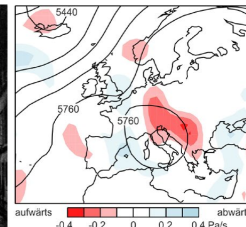
Abb. 5: (links) Hochwasser am 14. Juni 1910 in Bern (Hinkender Bot), (Mitte) Rekonstruktion des Wetters über Europa in 20CR (geopotentielle Höhe und Vertikalbewegung auf 500 hPa) um 12 UTC, (rechts) stündlicher Niederschlag über der Schweiz um 15 UTC im Downscaling mit WRF (Daten von Peter Stucki, Universität Bern).
