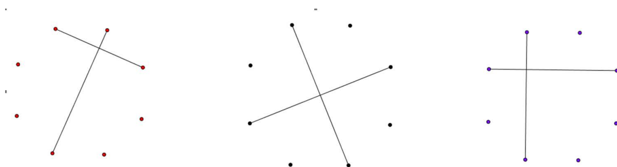
Image 1 : diverses perpendiculaires trouvées
