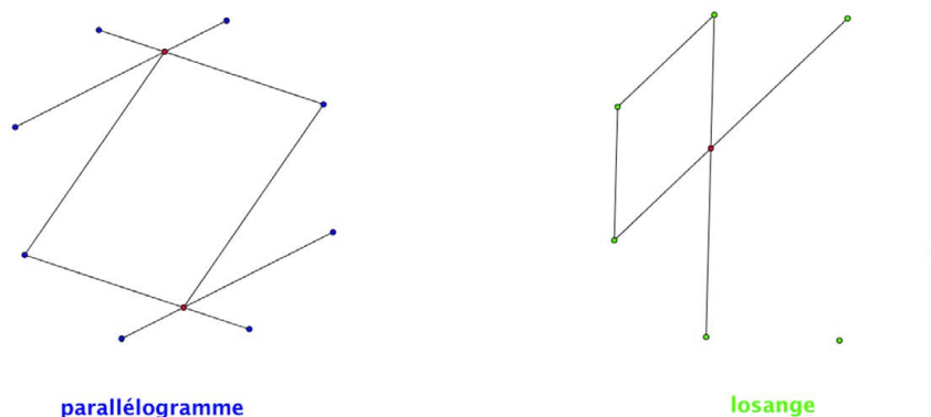
Image 7 : exemples de parallélogramme et de losange
