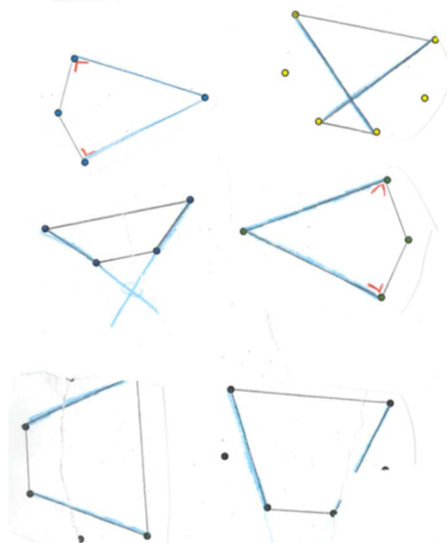
Image 6 : Erreurs sur le parallélisme (en bleu)
