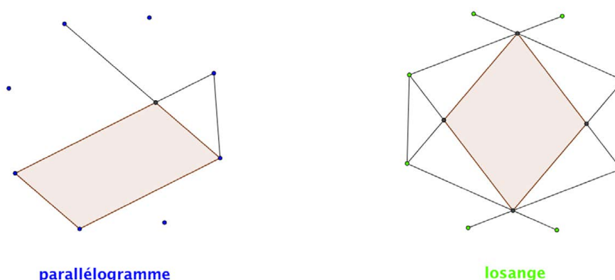
Image 8 : autres exemples de parallélogramme et de losange
