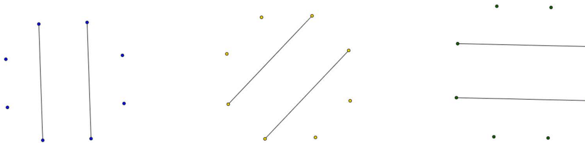
Image 3 : parallèles dans l'octogone régulier
